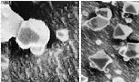
Kryształki suchego lodu ( \text{CO}_2 )
