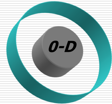
Kropka kwantowa – „sztuczny atom”
